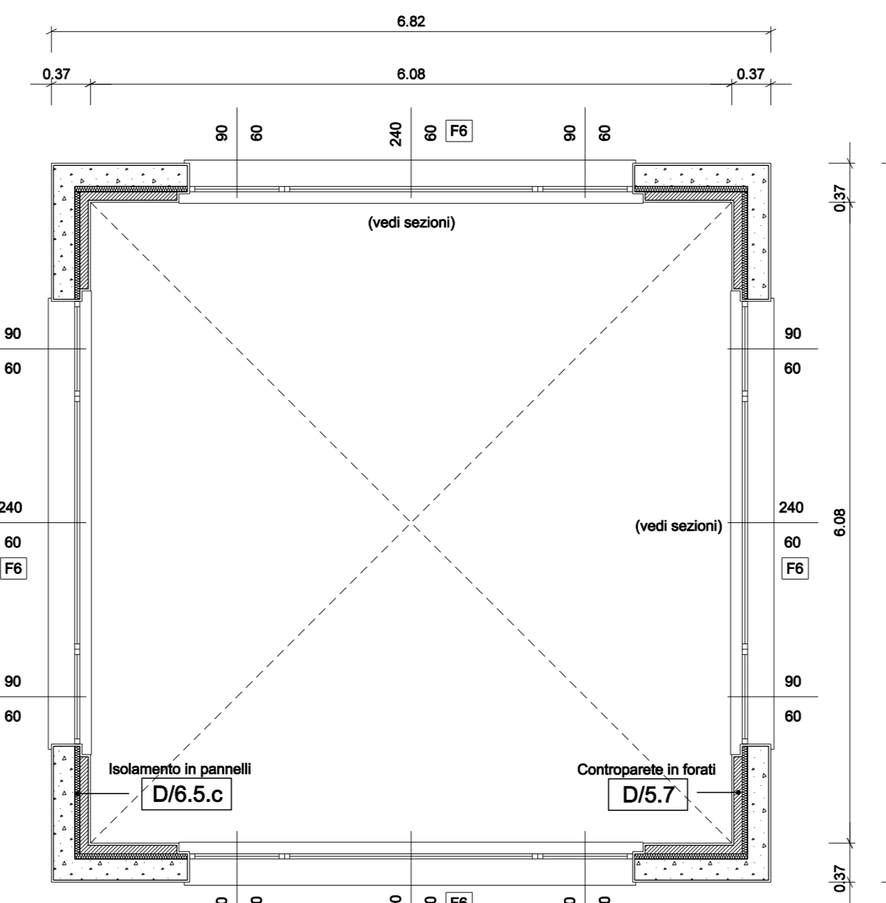
PARTICOLARE A QUOTA +3.50
