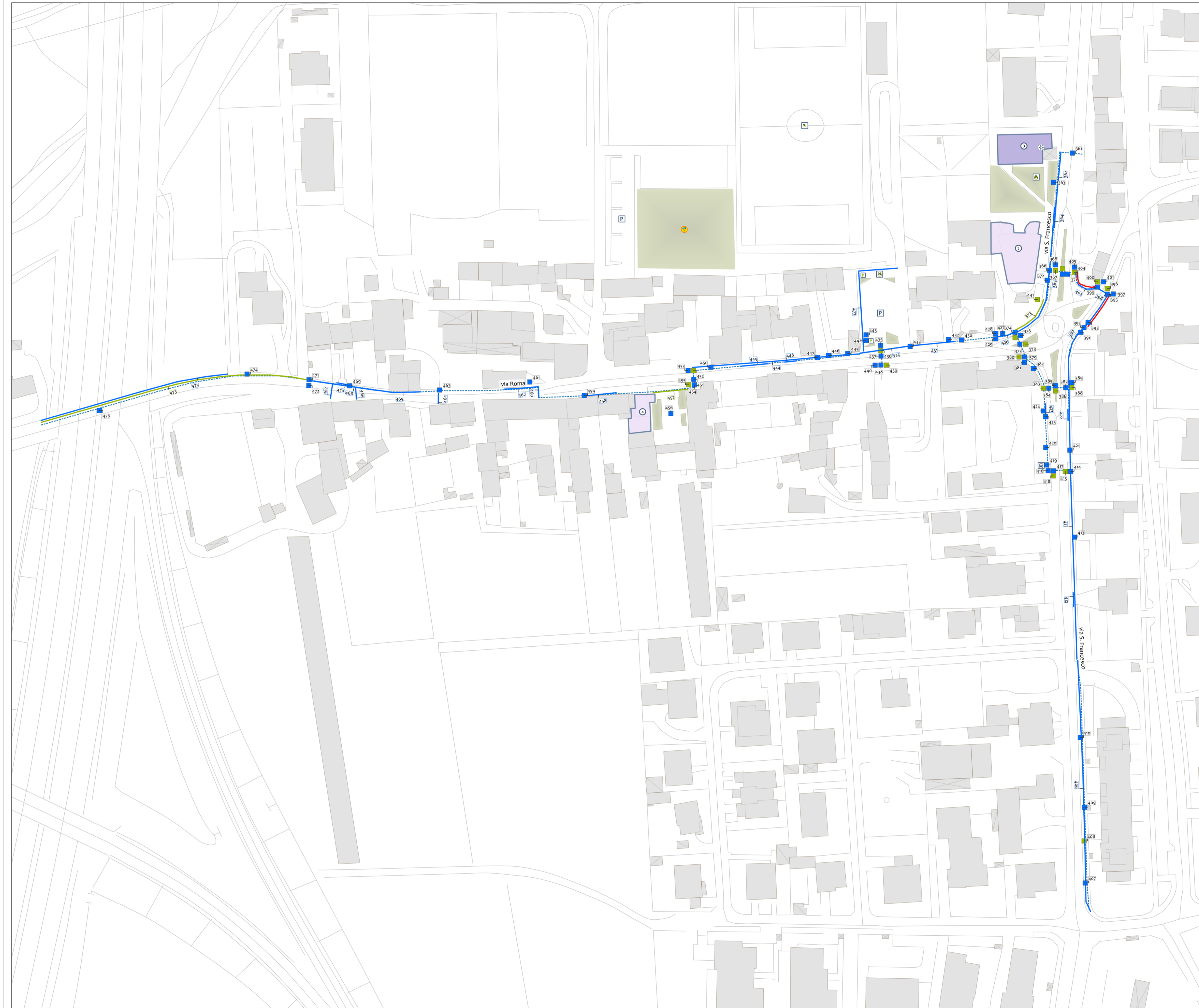
PLANIMETRIA_Branco scala 1:800
