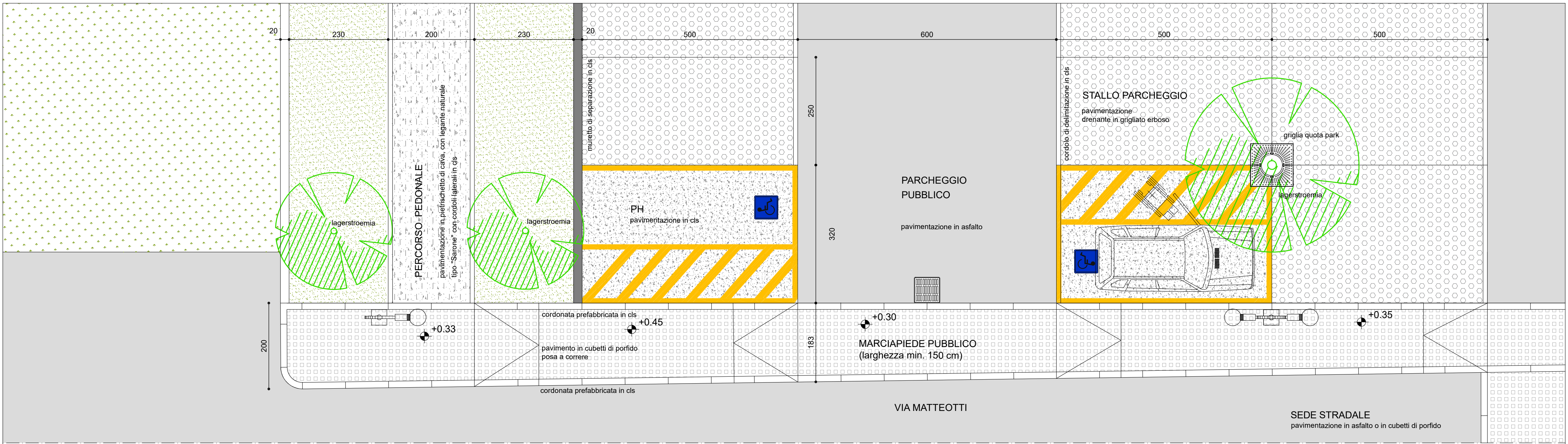
PARTICOLARE VIABILITA' PUBBLICA E PARCHEGGI - Scala 1:50
